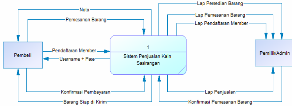
Gambar 4. Diagram Kontek Sistem E-Commerce UKM Produk Sasirangan Sumber : Diolah, 2015
