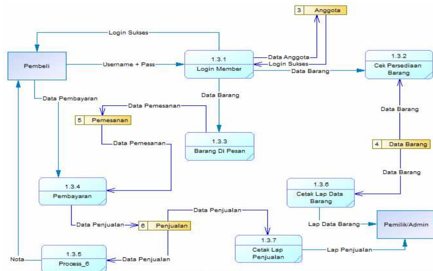
Gambar 6. DFD Level 2 Sumber : Diolah, 2016
