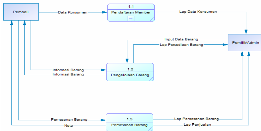
Gambar 5. DFD Level 1 Sumber : Diolah, 2016
