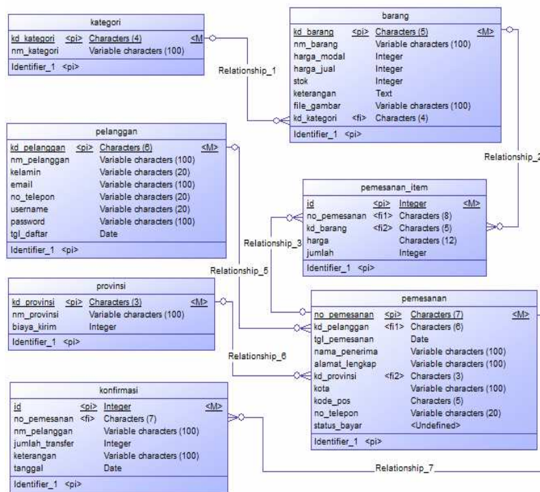
Gambar 7. Diagram ERD Sumber : Diolah, 2016
