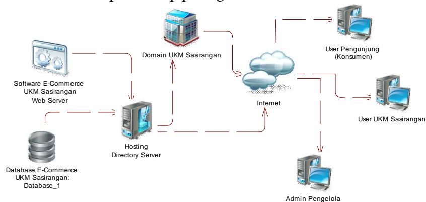
Gambar 3. Arsitektur Sistem E-Commerce UKM Produk Sasirangan Sumber : Diolah, 2016
