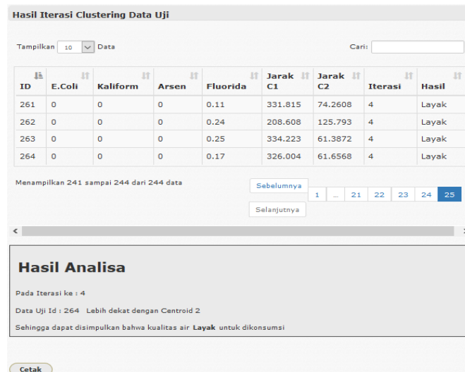
Gambar 7 Hasil Perhitungan K-Means Sampai Iterasi ke-4
