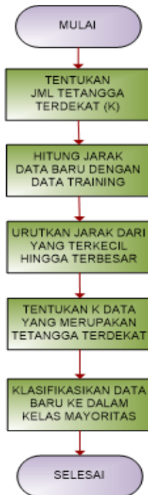
Gambar 1 Diagram Alir Metode KNN
