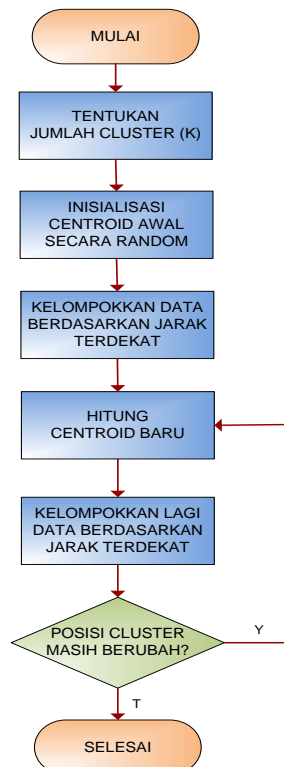
Gambar 2 Diagram Alir Metode K-Means
